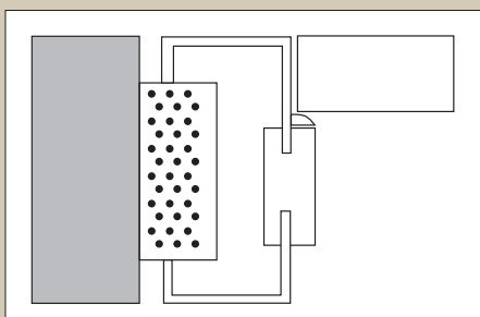
Türblatt stumpf einschlagend, Zarge flächenbündig, entsprechendes Wandöffnungsmaß muss bereits bei der Planung berücksichtigt werden.
