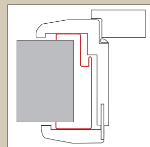
Türblatt gefälzt. Zarge bombiert 80 mm. Renovierungselement Stahlzargenummantelung.
