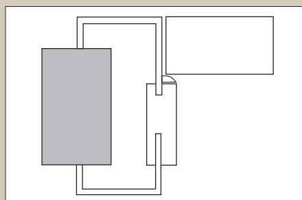
Türblatt stumpf einschlagend, Zarge eckig. Türblatt und Zarge flächenbündig.
