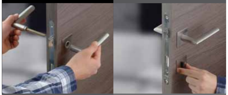
Türgriffe zusammenstecken
